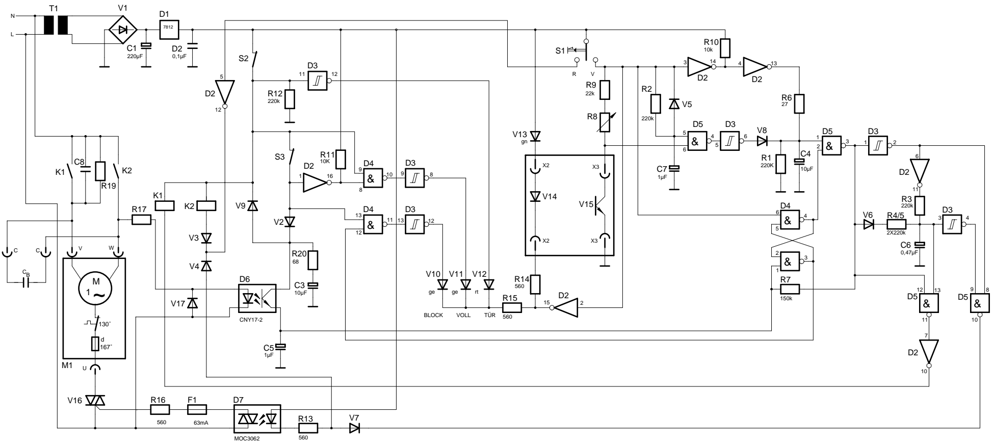
Stromlaufplan 2350 B schema de circuit électrique 2350 B wiring diagram 2350 B
